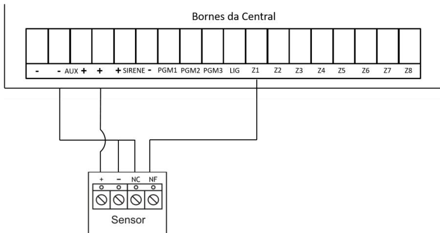
Figura 7 - Conexão do Sensor Sem RFL
