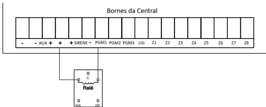
Figura 5 - Conexão do Borne PGM1
