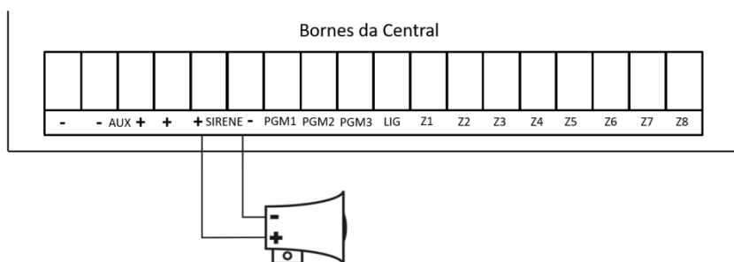
Figura 4 - Conexão da Sirene
