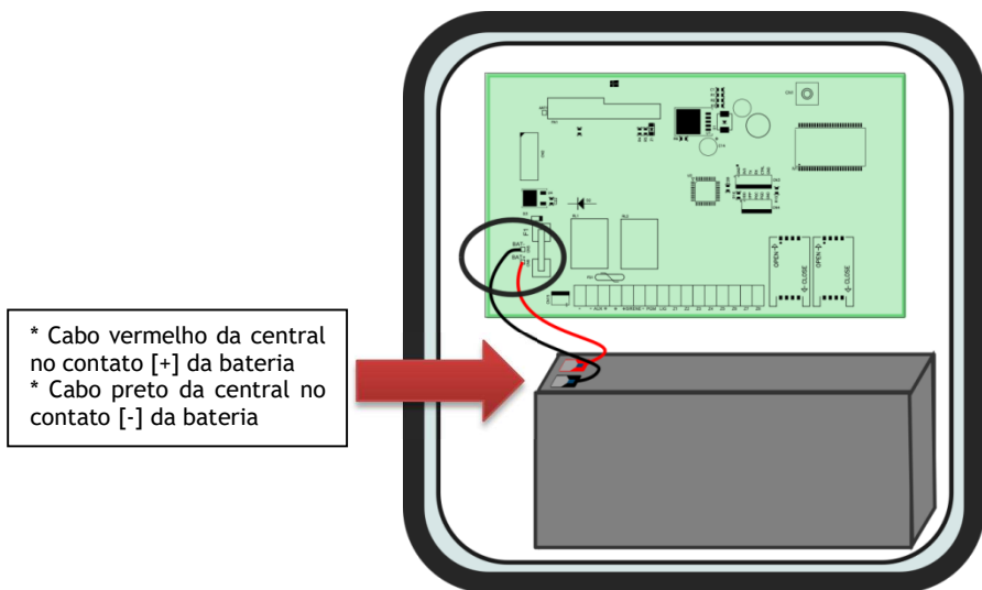
Figura 9 - Conexão da Bateria
