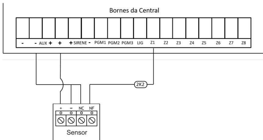
Figura 6 - Conexão do Sensor Com RFL
