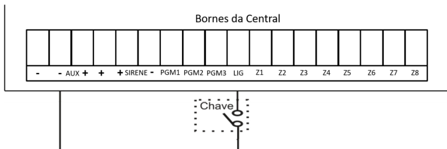
Figura 8 - Conexão do Borne LIG
